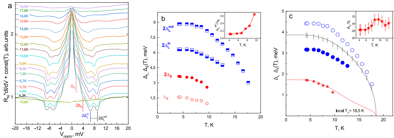
Рис. 4. (а) Температурная эволюция ДП-спектра андреевского SnS-контакта на основе \text{BaFe}_{1.93}\text{Ni}_{0.07}\text{As}_2 . Динамическая поводимость при T = 4.3 К и T = 19.6 К, по вертикали нормированная на своё значение при eV \gg 2\Delta(0) , совпадает, что доказывает неизменность нормального сопротивления контакта выше и ниже T_c . Спектры для остальных значений температур 4.4 \leq T \leq 18.5 К вручную смещены по вертикали для удобства анализа. Вертикальными линиями указано положение особенностей СГС от большой и малой СП-щелей при T = 4.3 К. (б) Температурные зависимости положений особенностей на dI/dV спектрах, обозначенных на графике (а), размер символа соответствует величине погрешности измерений. На вставке построено отношение среднего значения амплитуды большой СП-щели \Delta_L^{eff} = (\Delta_L^{out} + \Delta_L^{in})/2 к малой \Delta_S от температуры. (с) Температурные зависимости СП-щелей по данным (а, б). Приведены результаты расчета в рамках двухщелевой модели Москаленко и Сула [27, 28], в качестве температурной зависимости большой СП-щели взята \Delta_L^{eff}(T) . На вставке показано, что параметр анизотропии большой СП-щели A_L = 100\% \cdot [1 - \Delta_L^{in}/\Delta_L^{out}] слабо зависит от температуры и сохраняется примерно равным A_L \approx (30 \pm 5)\% .
